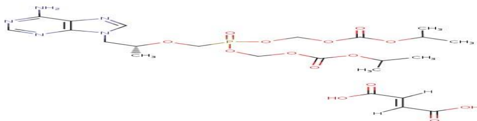
Fig.1 Tenofovir Disoproxil Fumarate
